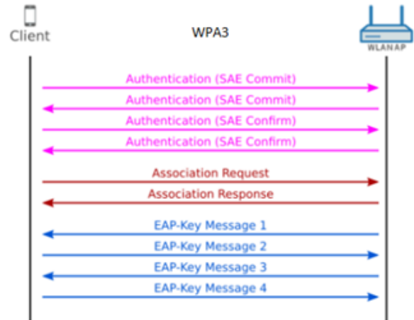
Рис 3. Схема підключення WPA3
