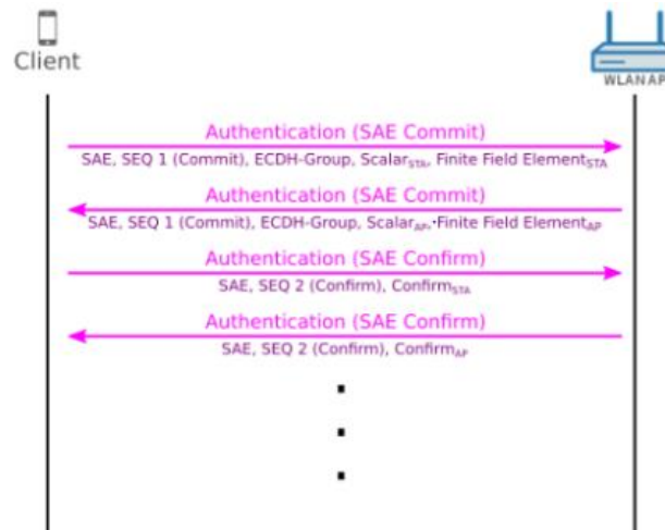
Рис 4. Повідомлення автентифікації WPA3
